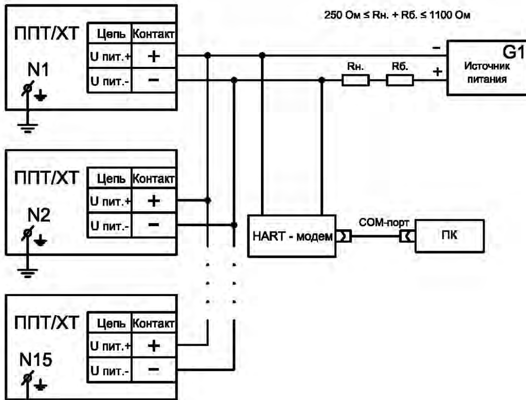
Рисунок Ж.22 – Схема подключения ППТ/ХТ-W к сопротивлению нагрузки R_n , сопротивлению R_b , источнику питания G1, HART-модему и ПК в многоточечном режиме
