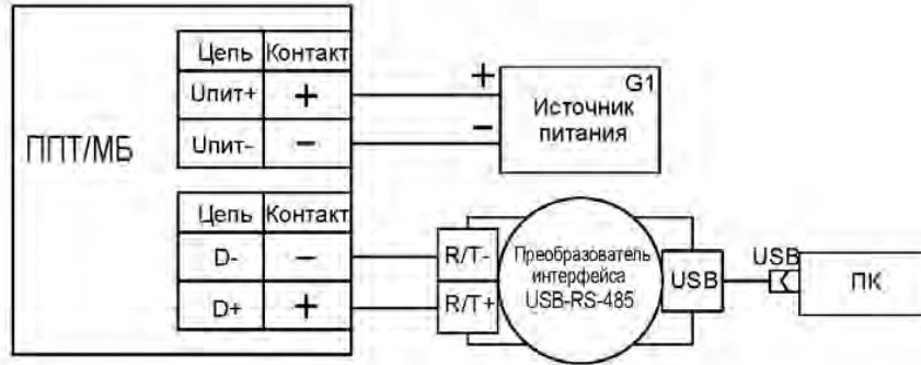
Рисунок 2.20 – Схема подключения ППТ/МБ к источнику питания G1, преобразователю интерфейса USB-RS485 и ПК
