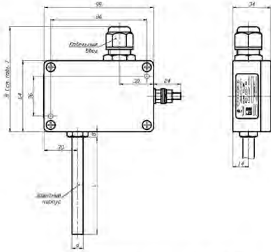
ППТС (ППТСК, ППТП) с головкой типа «Г8/1»: Г8/1/Оп, Г8/1/Ек1 (материал головки - алюминиевый сплав)
