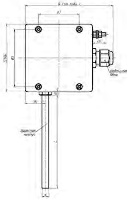
ППТС (ППТСК, ППТП) с головкой типа «Г8/2Н», Г8/2Н/Оп, Г8/2Н/Ек (материал головки - нержавеющая сталь)
