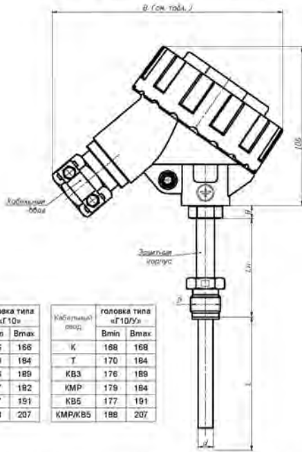
ПТС (ПТСК, ПТП) с головкой типа «Г10/У»: Г10/У/Оп, Г10/У/Ехд, Г10/У/Ех, Г10/У/Ехд (материал головки - алюминиевый сплав)
