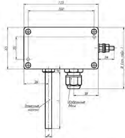
ППТС (ППТСК, ППТП) с головкой типа «Г8/1ПРТУ»: Г8/1ПРТУ/Оп, Г8/1ПРТУ/Ек1 (материал головки - алюминиевый сплав)
