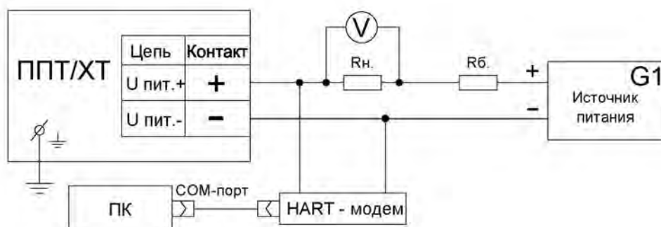
Рисунок Ж.1 – Схема подключения ППТ/ХТ-В к источнику питания G1, сопротивлению нагрузки Rн., сопротивлению Rб., вольтметру V и ПК
