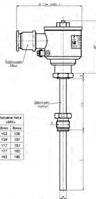
Рисунок Г.8 - Общий вид ПТС (ПТСК, ПТП) с головками типов «Г10», «Г10/У», «М(D)», «МН» и ПТС/ИНД (ПТСК/ИНД, ПТП/ИНД) с головками типов «Г11», «Г11/У»
