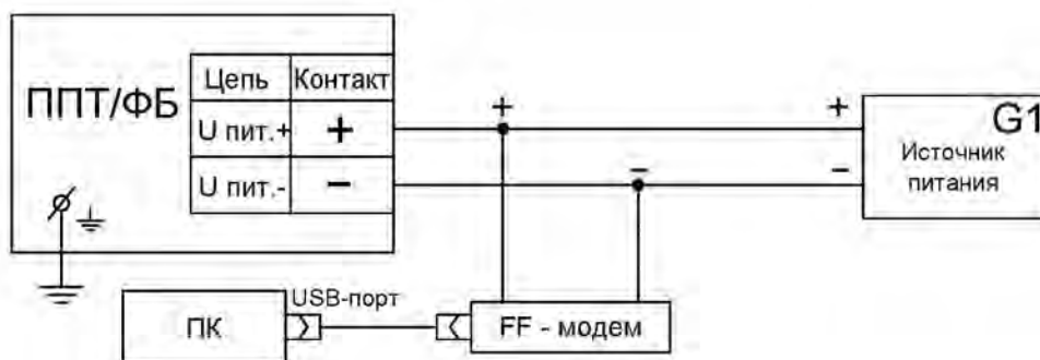
Рисунок С.6 – Схема соединения ИП/ФБ, ИП/ЛБ с FF-модемом и ПК с внешним источником питания G1
