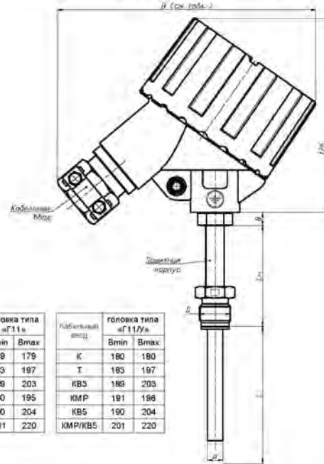
ПТС/ИНД (ПТСК/ИНД, ПТП/ИНД) с головкой типа «Г11/У»: Г11/У/Оп, Г11/У/Ехд, Г11/У/Ех, Г11/У/Ехд (материал головки - алюминиевый сплав)
