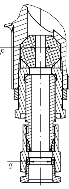
Кабельный ввод КВЗ с поддержанием непрерывности цепи заземления
