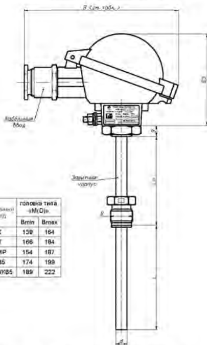
Рисунок Г.8 - Общий вид ПТС (ПТСК, ПТП) с головками типов «Г10», «Г10/У», «М(D)», «МН» и ПТС/ИНД (ПТСК/ИНД, ПТП/ИНД) с головками типов «Г11», «Г11/У»
