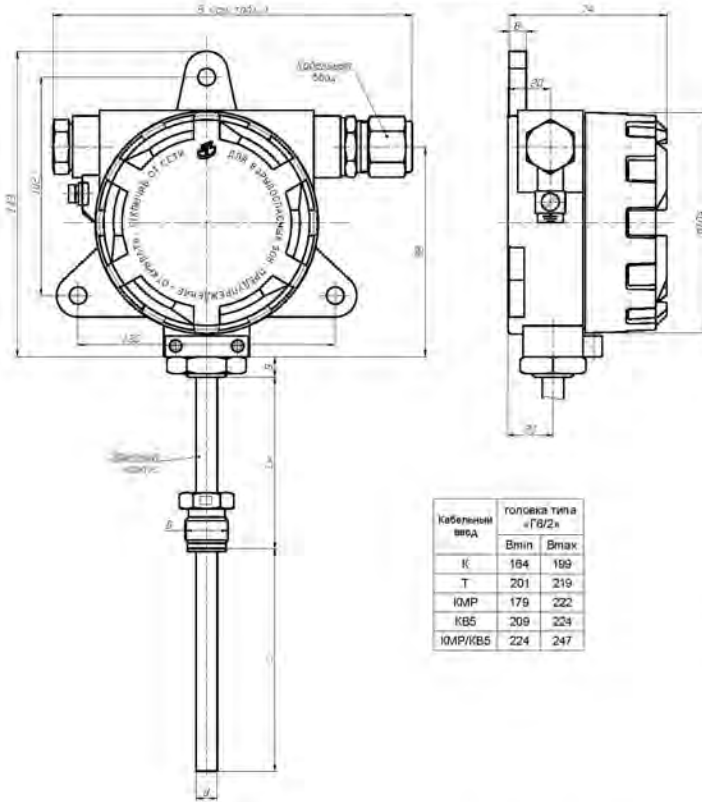
ППТС (ППТСК, ППТП) с головкой типа «Г6/2»: Г6/2/Оп, Г6/2/Ехд, Г6/2/Ех, Г6/2/Ехд (материал головки - алюминиевый сплав)
