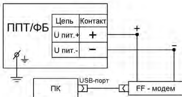
Рисунок С.7 – Схема соединения ИП/ФБ, ИП/ЛБ с FF-модемом и ПК с питанием от FF-модема
