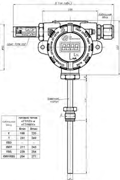
Рисунок Г.3 - Общий вид ППТС (ППТСК, ППТП) с головками типов «ГБ/1», «ГБ/1М», «ГБ/1У», «ГБ/1МУ» и ППТС/ИНД (ППТСК/ИНД, ППТП/ИНД) с головками типов «Г7/1», «Г7/1М», «Г7/1У», «Г7/1МУ»
