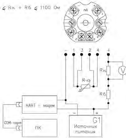
Рисунок С.2 – Схема подключения к ИП/ХТ-W магазина сопротивлений Rчэ, имитирующего сопротивление ЧЭ, источника питания G1, сопротивления нагрузки Rн., вольтметра V, FSK-модема и ПК
