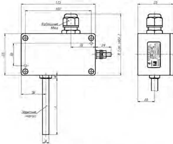
ППТС (ППТСК, ППТП) с головкой типа «Г8/1У»: Г8/1У/Оп, Г8/1У/Ек1 (материал головки - алюминиевый сплав)
