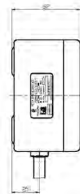
ППТС (ППТСК, ППТП) с головкой типа «Г8/2Н», Г8/2Н/Оп, Г8/2Н/Ек (материал головки - нержавеющая сталь)
