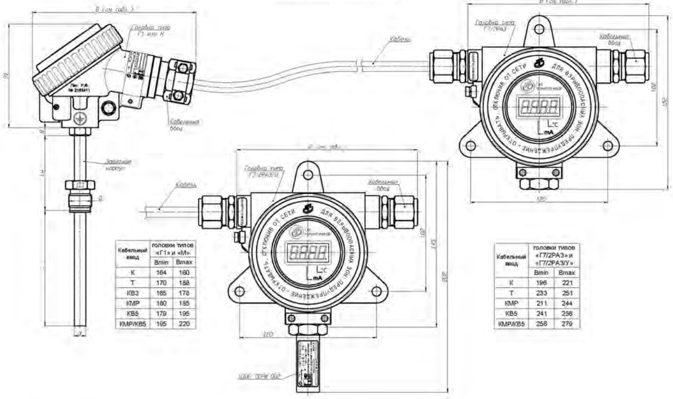
Рисунок Г.9в - Общий вид ПТТСК с головками типов «Г6/2РА3/Г1», «Г6/2РА3/У/Г1», «Г6/2РА3/М», «Г6/2РА3/У/М» и ПТТСК/ИНД с головками типов «Г7/2РА3/Г1», «Г7/2РА3/У/Г1», «Г7/2РА3/М», «Г7/2РА3/У/М»
