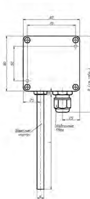
ППТС (ППТСК, ППТП) с головкой типа «Г9ПРТ», Г9ПРТ/Оп, Г9ПРТ/Ек (материал головки - поликарбонат)
