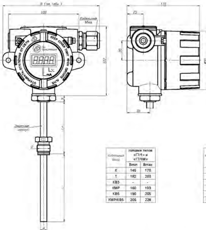
Рисунок Г.3 - Общий вид ППТС (ППТСК, ППТП) с головками типов «ГБ/1», «ГБ/1М», «ГБ/1У», «ГБ/1МУ» и ППТС/ИНД (ППТСК/ИНД, ППТП/ИНД) с головками типов «Г7/1», «Г7/1М», «Г7/1У», «Г7/1МУ»
