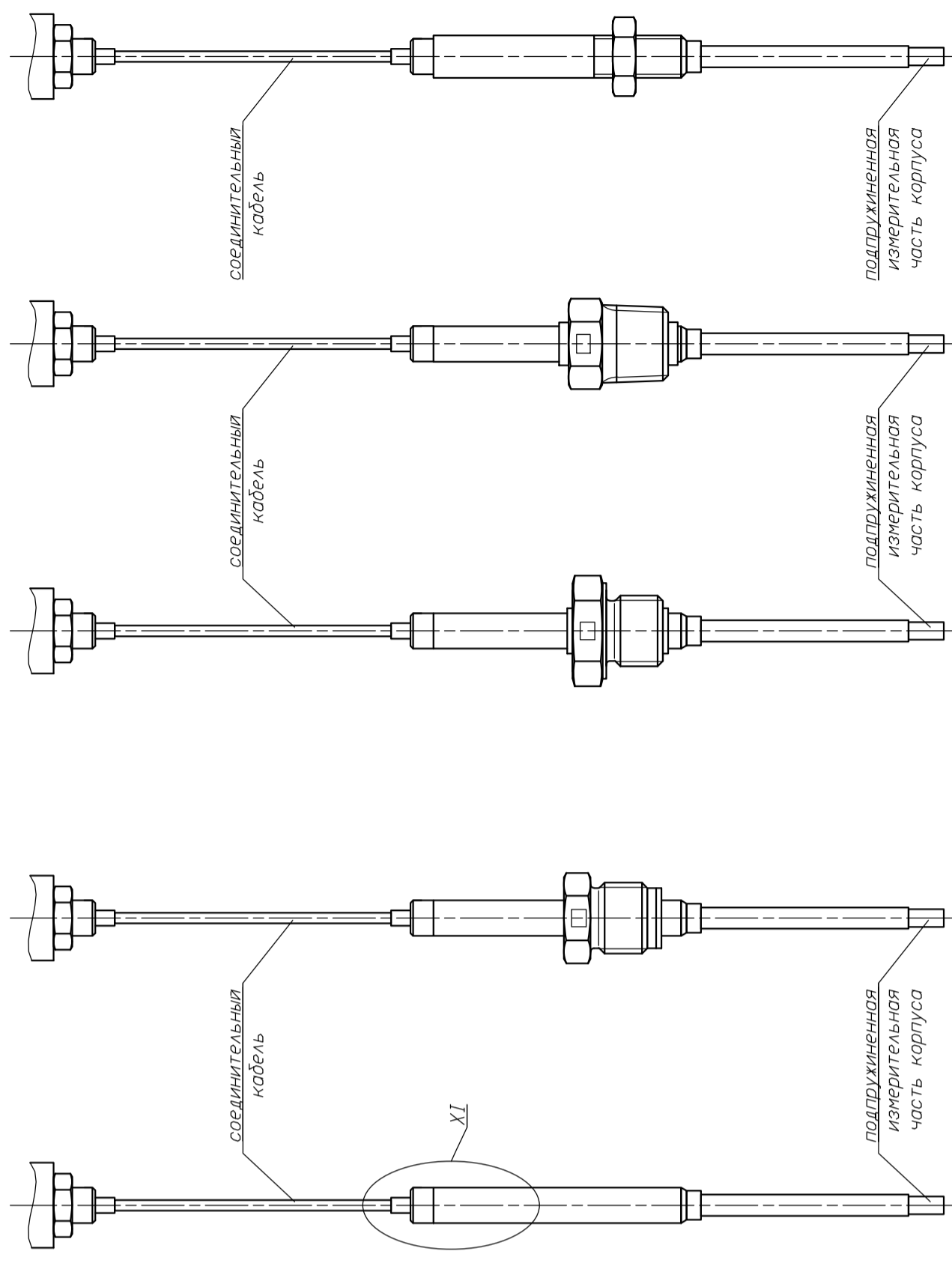
Варианты исполнения защитного корпуса с соединительным кабелем на основе гибких кабелей типов КНМСН, КНМСМ или КТМС и подпружиненной измерительной частью
