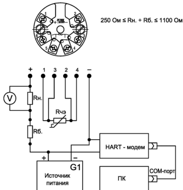
Рисунок С.3 – Схема подключения к ИП/ХТ-У, ИП/ХТ-РР, ИП/ХТ-РР1, ИП/ХТ-Е магазина сопротивлений R_{\text{чэ}} , имитирующего сопротивление R_{\text{чэ}} , источника питания G1 , сопротивления нагрузки R_{\text{н.}} , вольтметра V , FSK-модема и ПК
