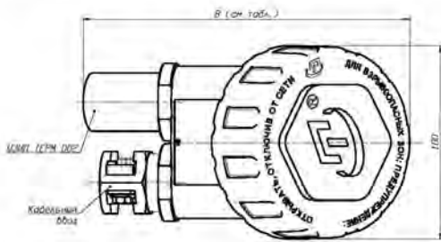
ПТС (ПТСК, ПТП) с головкой типа «М(D)»: М(D)/Оп, М(D)/Ех (материал головки - алюминиевый сплав)
