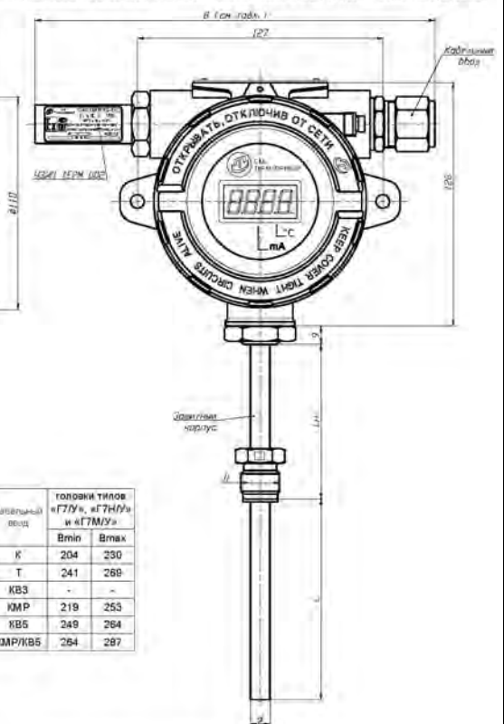
Рисунок Г.2 - Общий вид ППТС (ППТСК, ППТП) с головками типов «Г6», «Г6Н», «Г6М», «Г6У», «Г6НУ», «Г6МУ» и ППТС/ИНД (ППТСК/ИНД, ППТП/ИНД) с головками типов «Г7», «Г7Н», «Г7М», «Г7У», «Г7НУ», «Г7МУ»
