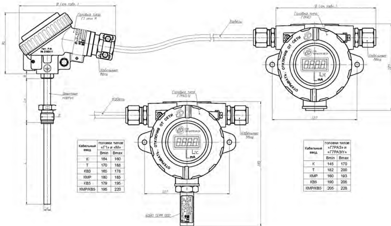
Рисунок Г.9 - Общий вид ПТТСК с головками типов «Г6РАЗ/Г1», «Г6РАЗ/У/Г1», «Г6РАЗ/М», «Г6РАЗ/У/М» и ПТТСК/ИНД с головками типов «Г7РАЗ/Г1», «Г7РАЗ/У/Г1», «Г7РАЗ/М», «Г7РАЗ/У/М»
