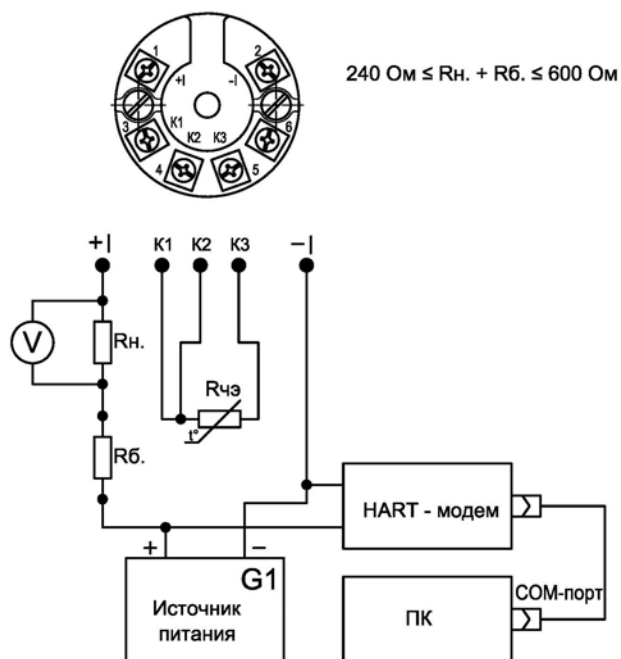
Рисунок С.4 – Схема подключения к ИП/ХТ-Э1 магазина сопротивлений R_{\text{чэ}} , имитирующего сопротивление R_{\text{чэ}} , источника питания G1 , сопротивления нагрузки R_{\text{н.}} , вольтметра V , FSK-модема и ПК
