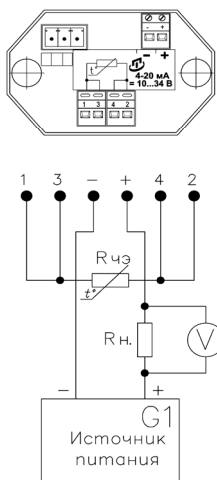
Рисунок С.1 – Схема подключения к ИП/МП магазина сопротивлений R_{чэ} , имитирующего сопротивление R_{чэ} , источника питания G1 , сопротивления нагрузки R_n и вольтметра V
