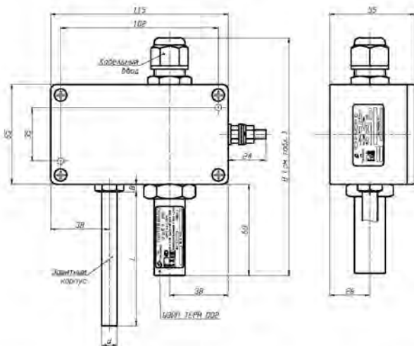
Рисунок Г.6 - Общий вид ППТС (ППТСК, ППТП) с головками типов «Г8», «Г8ПРТ», «Г8/1», «Г8/1ПРТ», «Г8/1У», «Г8/1ПРТУ»
