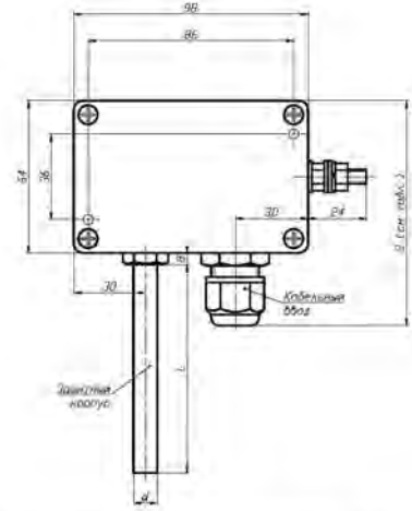
ППТС (ППТСК, ППТП) с головкой типа «Г8/1ПРТ»: Г8/1ПРТ/Оп, Г8/1ПРТ/Ек1 (материал головки - алюминиевый сплав)
