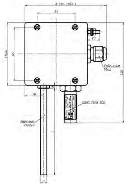
ППТС (ППТСК, ППТП) с головкой типа «Г8/2Н/У», Г8/2Н/У/Оп, Г8/2Н/У/Ек (материал головки - нержавеющая сталь)
