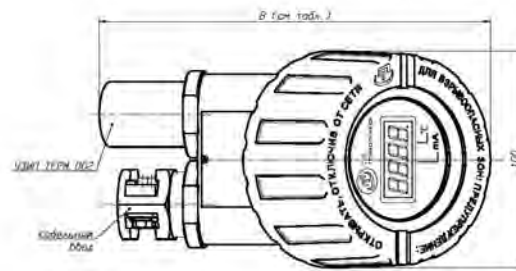
ПТС (ПТСК, ПТП) с головкой типа «МН»: МН/Оп, МН/Ех (материал головки - нержавеющая сталь)
