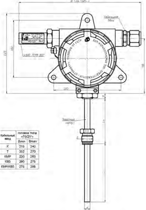
ППТС (ППТСК, ППТП) с головкой типа «Г6/2У»: Г6/2У/Оп, Г6/2У/Ехд, Г6/2У/Ех, Г6/2У/Ехд (материал головки - алюминиевый сплав)
