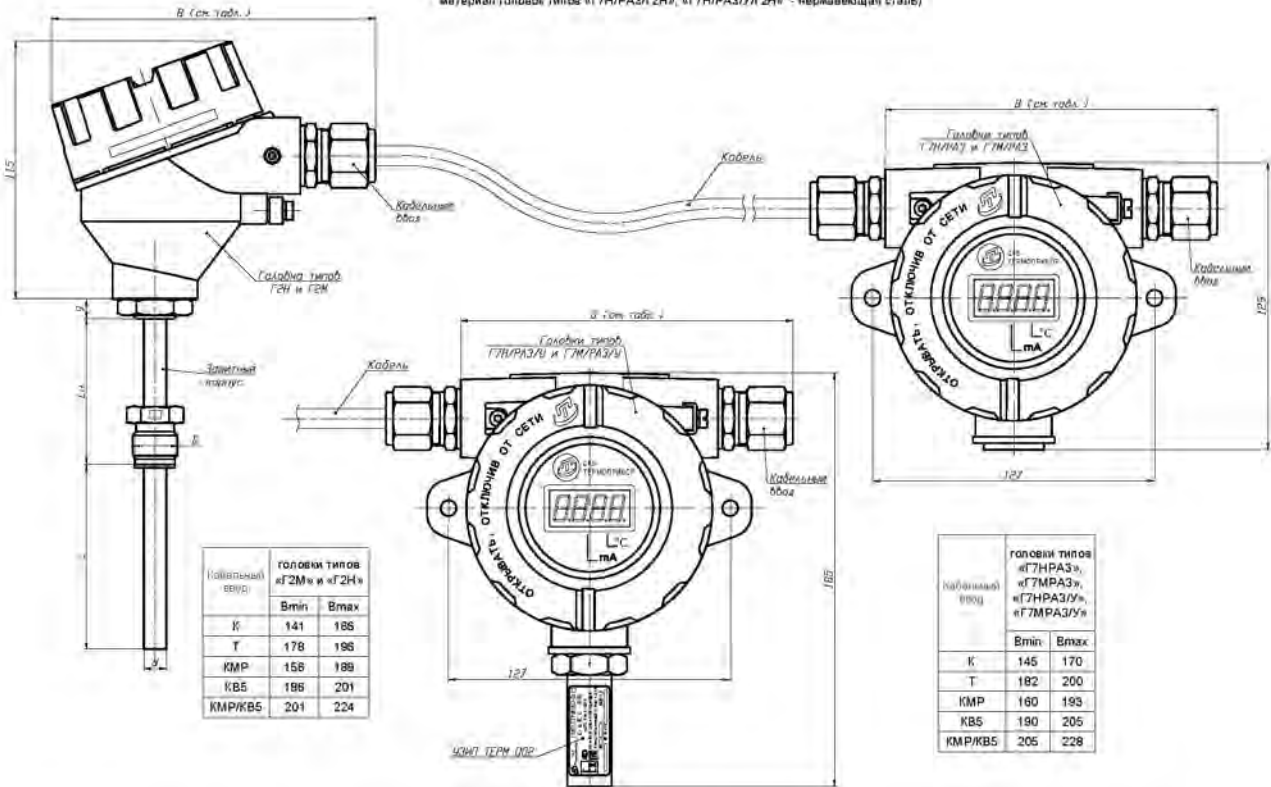
Рисунок Г.10 - Общий вид ППТСК с головками типов «Г6Н/РА3/Г2Н», «Г6М/РА3/Г2М», «Г6Н/РА3/УГ2Н», «Г6М/РА3/УГ2М» и ППТСК/ИНД с головками типов «Г7Н/РА3/Г2Н», «Г7М/РА3/Г2М», «Г7Н/РА3/УГ2Н», «Г7М/РА3/УГ2М»
